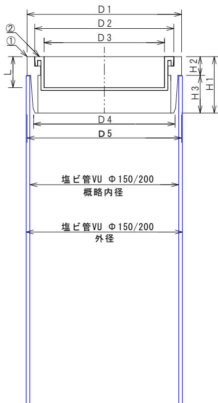
A-A' 断面図
