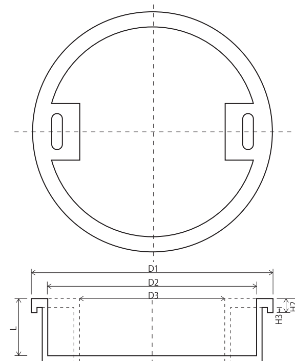
Φ250・300タイプ 寸法図
