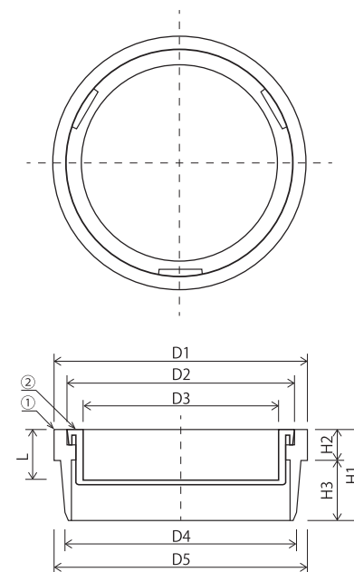
Φ150・200タイプ 寸法図
